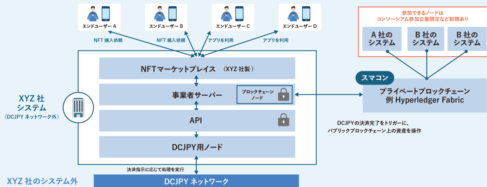
図2.9 想定システムモデル 3
