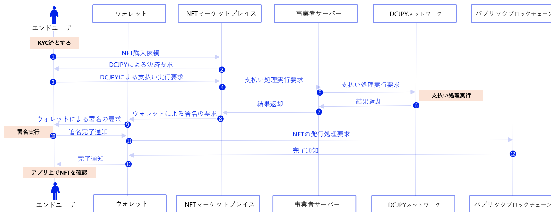
図2.8 想定システムモデル2のフロー例
