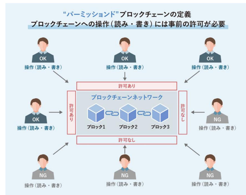
図2.4 パーミッションド分散台帳の概念
